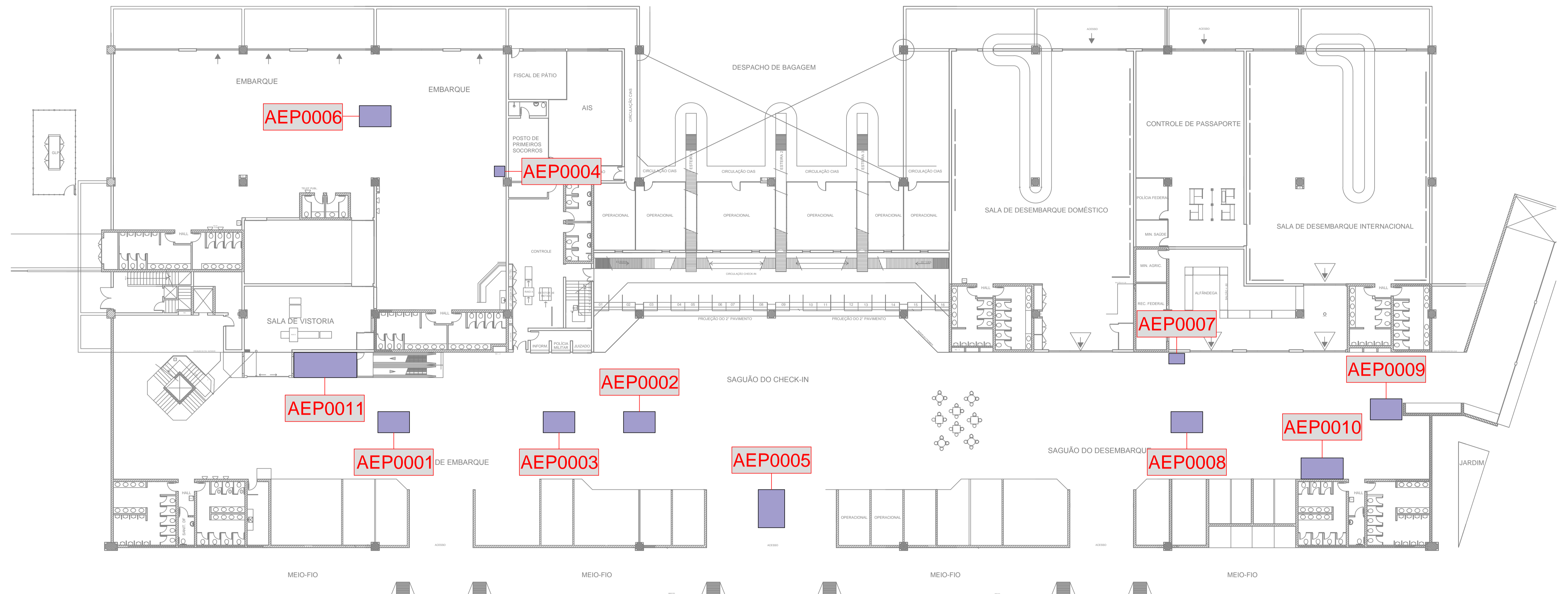
PLANTA BAIXA - PAVIMENTO TÉRREO ESCALA 1:350
